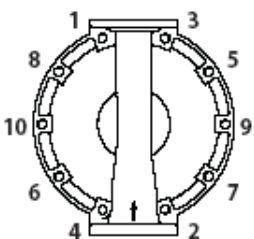
Последовательность затяжки болтов
