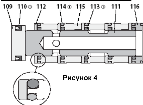
Главный воздушный клапан в разрезе
